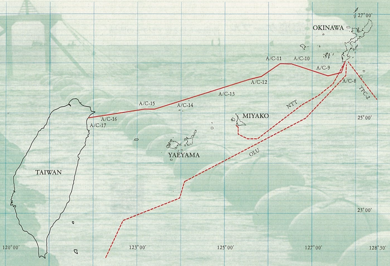
[Map] 出典：「沖縄・台湾間海底ケーブル建設記録」国際電信電話株式会社 1980年11月、16頁 [Photo] 沖縄側陸揚工事(KDD丸) 出典：「沖縄・台湾間海底ケーブル建設記録」国際電信電話株式会社 1980年11月、口絵
